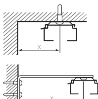
Tak samt väggmontage
